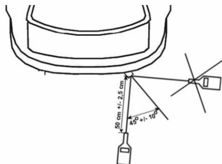
Fig 3e Skråstillet udstødningsrør.
