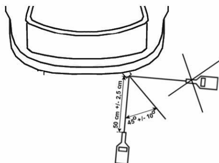
Fig 3e Skråstillet udstødningsrør.
